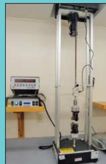
1,000 Lb. Con Tec Industries Model 951KBC-2000 Tensile Tester
